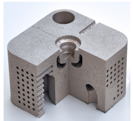
Kunststoffspritzgusseinsatz
